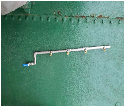
이중밸브 포함 완성된 세척기
