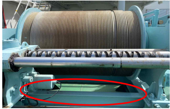
코어원치 프레임 4단 스프링클러 세척기 설치 Position
